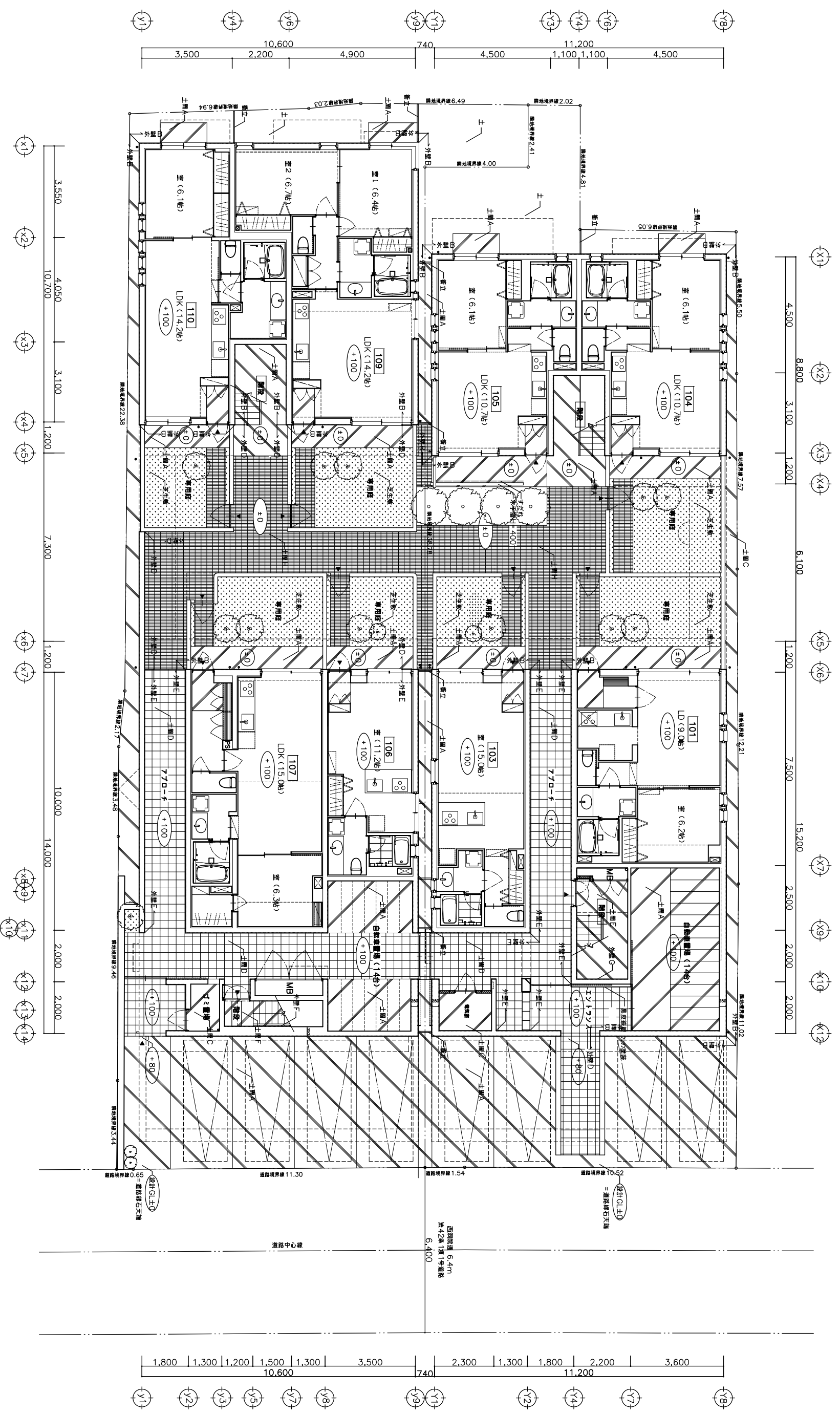
1階平面図 1/150
